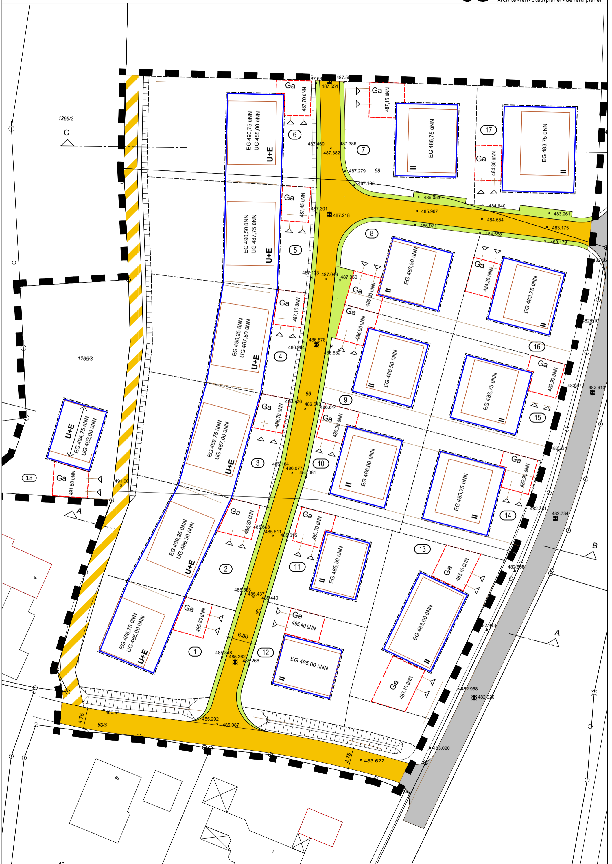
BEBAUUNGSPLAN "AM UNTERFELD, OBERORNAU" | HÖHENPLAN | M 1:500 | 10.03.2021
