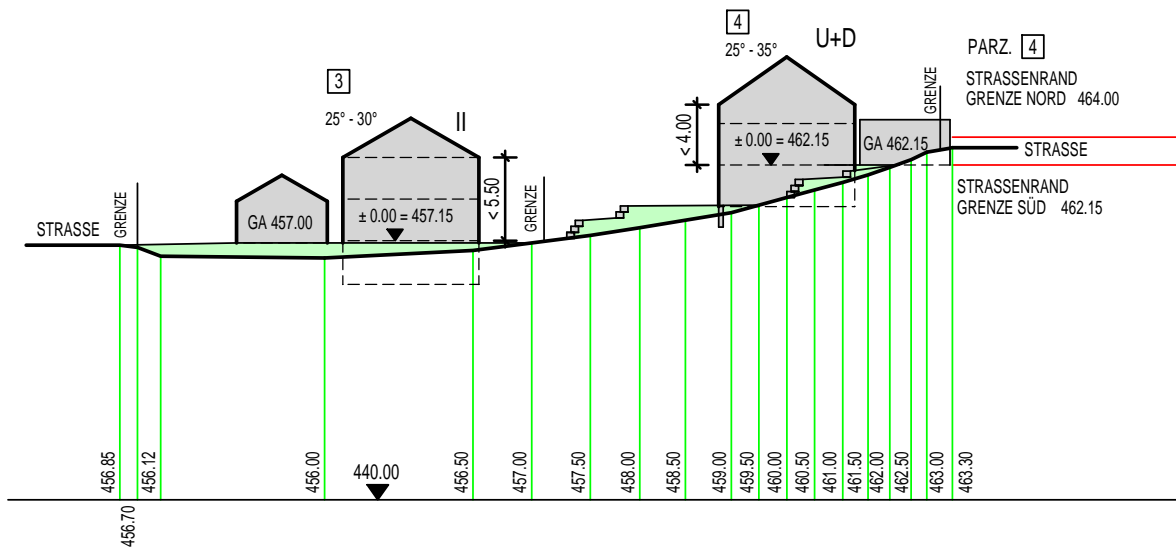
SCHNITT 2 - 2
